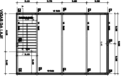
VIGAS DA LAJE Figura 1.20
