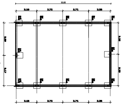
PLANTA DE FUNDAÇÃO - BLOCOS E BROCAS Figura 1.18
