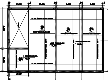
PLANO DA LAJE Figura 1.21
